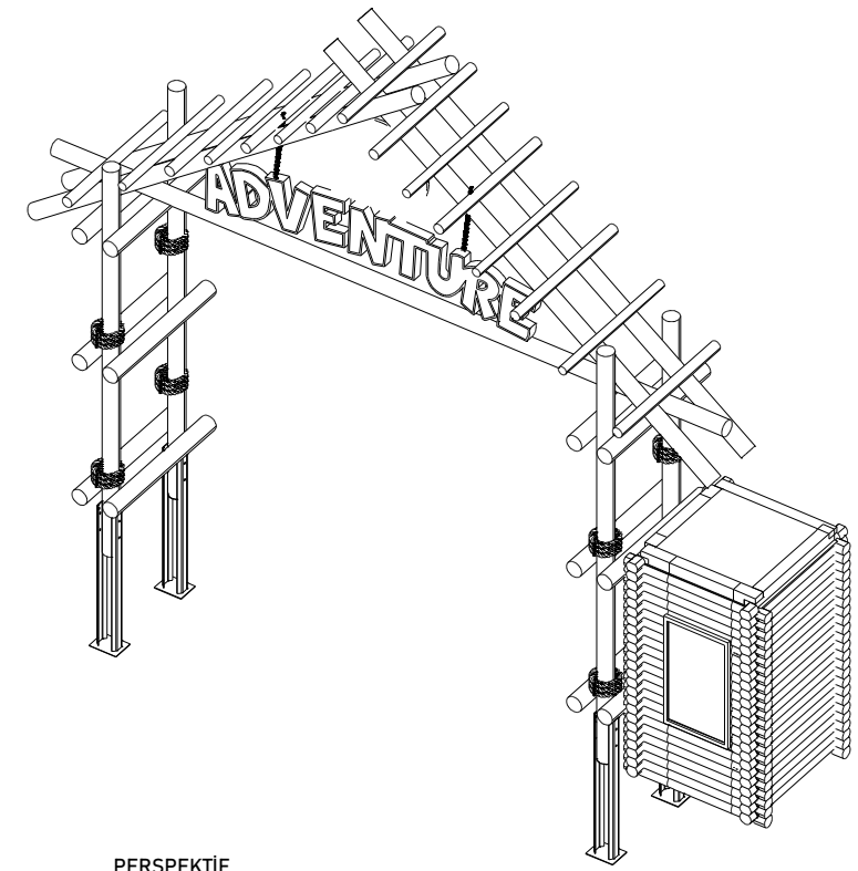
PERSPEKTİF
